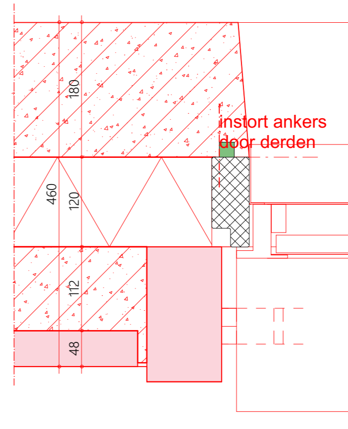
detail zijstijl
