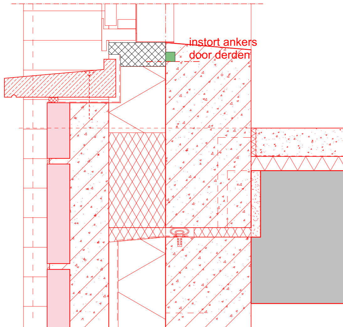
detail onderdorpel
