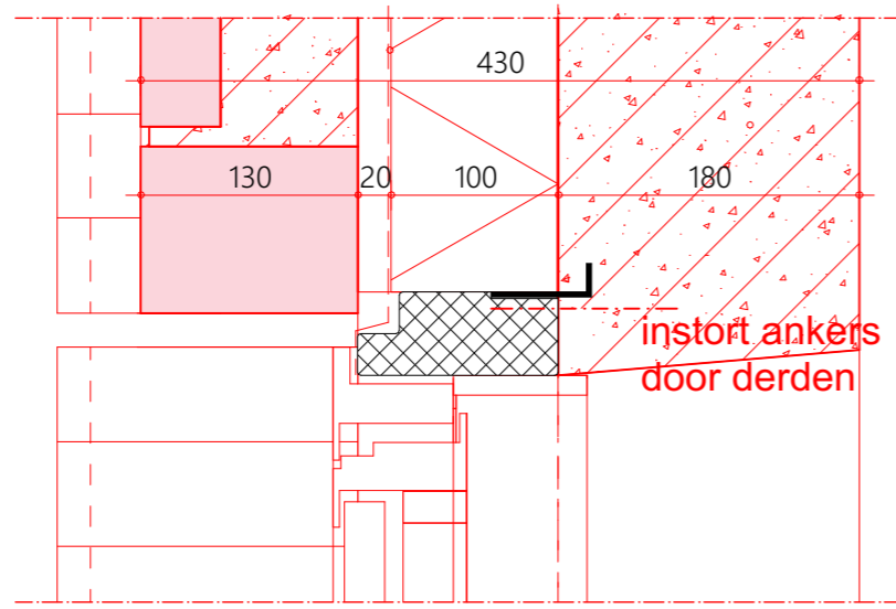
detail bovendorpel
